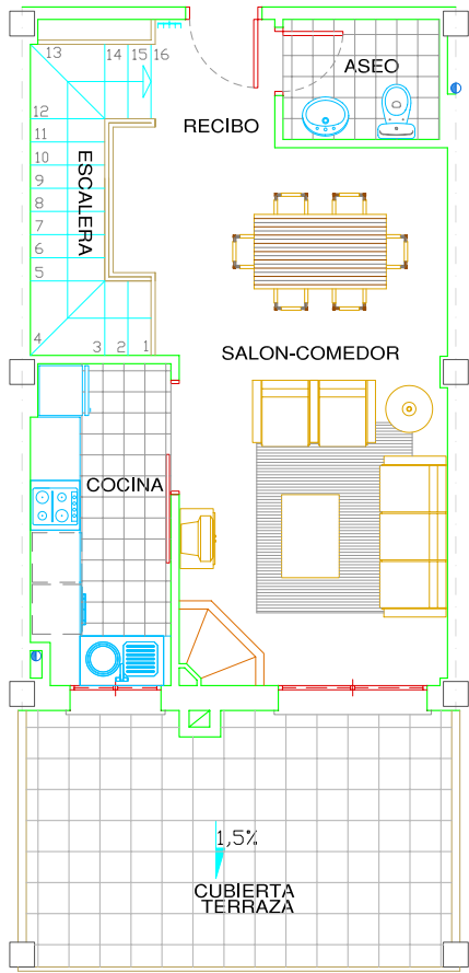
PLANTA 1ª
