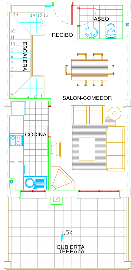
PLANTA 1ª
